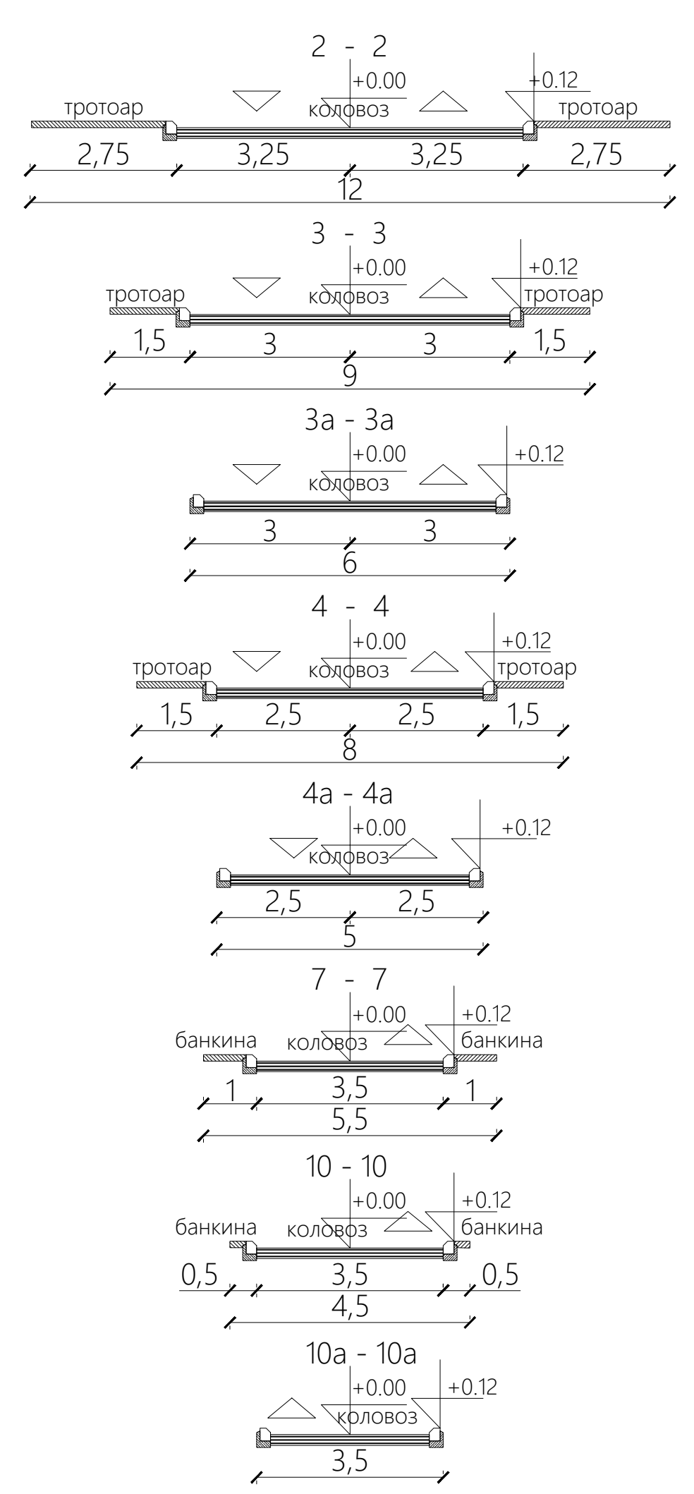
ПОПРЕЧНИ ПРОФИЛИ P 1:200
